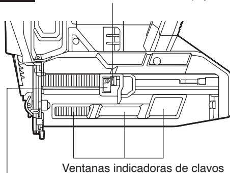
Fig. 5b Palanca de liberación del empujador
